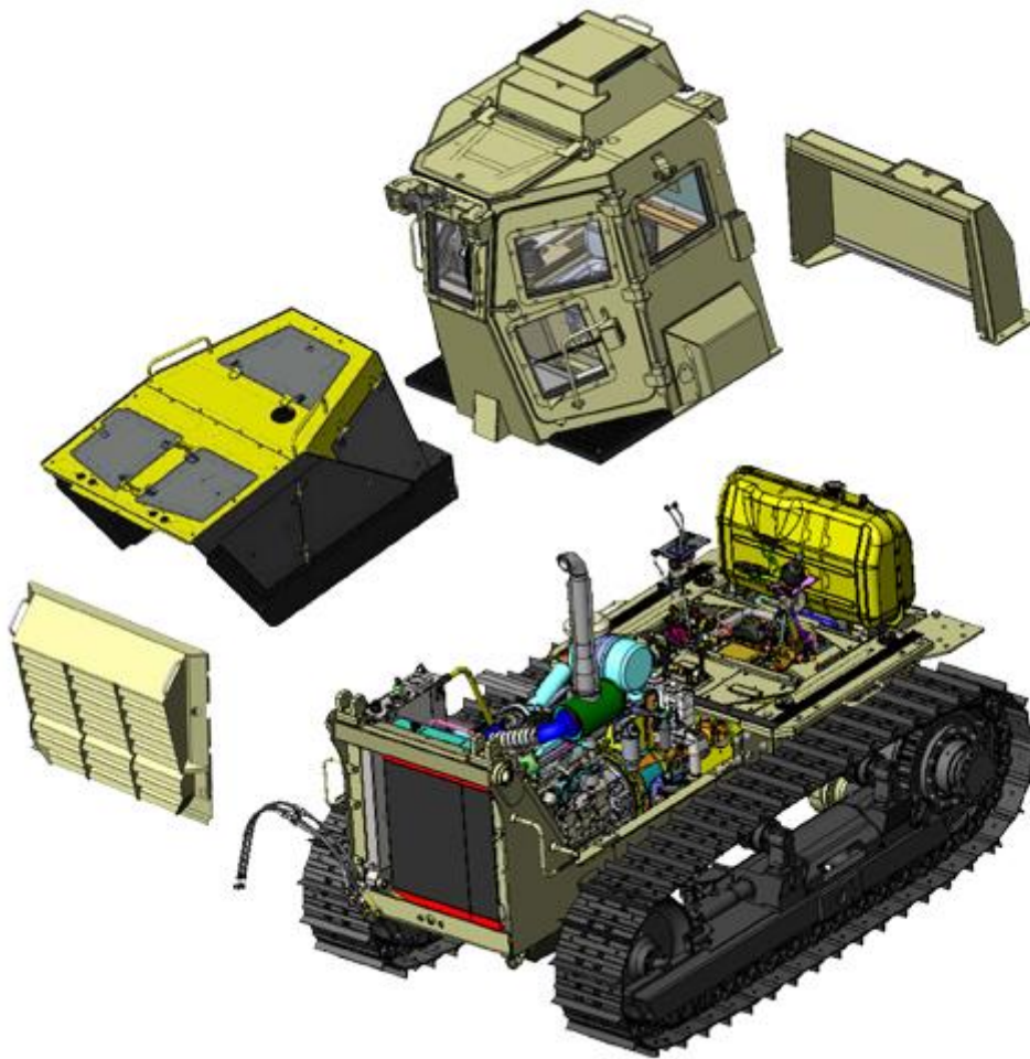
Рис. 2. Базовое шасси трактора Т10М2С/Т12С (серийное) и элементы специальной защиты (защита радиаторов, капот, кабина, защита топливного бака).
